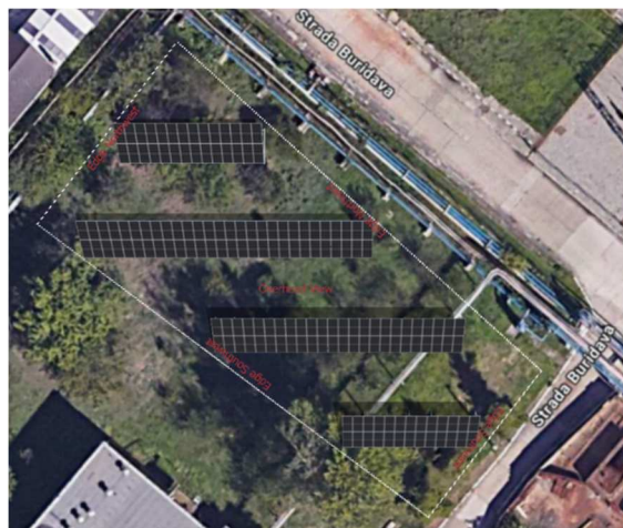
Fig. Zona 4 Panouri fotovoltaice
