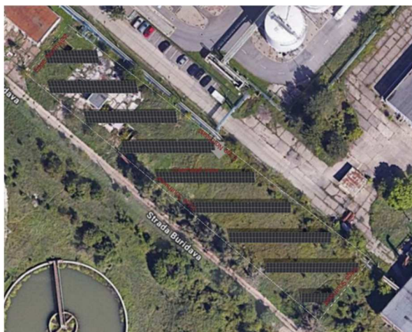
Fig. Zona 3 Panouri fotovoltaice
